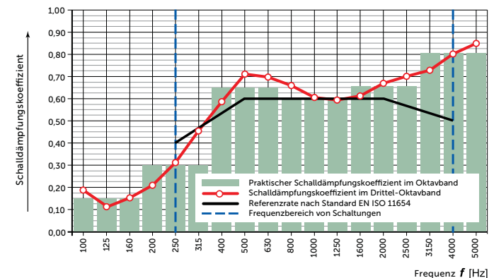
Praktischer Schalldämpfungskoeffizient nach Standard EN ISO 11654, \alpha_w : 0,60 Schalldämpfungs-kategorie nach EN ISO 11654: C
