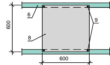
Befestigung von 600x600 Platten mit 4 Schrauben
