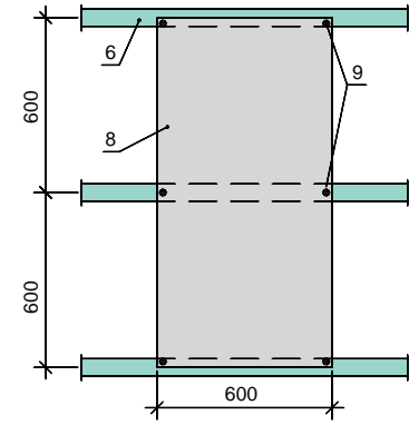
Befestigung von 600x1200 Platten mit 6 Schrauben
