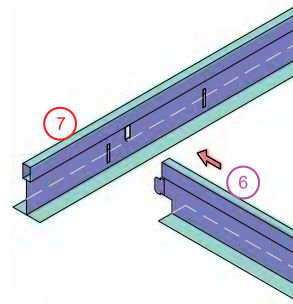
6 - Querprofil
