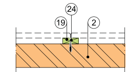
Befestigung von Holzlatten an der tragenden Wandkonstruktion
