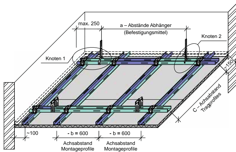
Montageabstand für Profile - 600 mm
