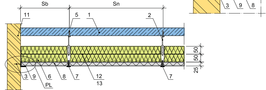
Abschnitt B1-B1, Profilanordnung für 595x595 mm Platten
