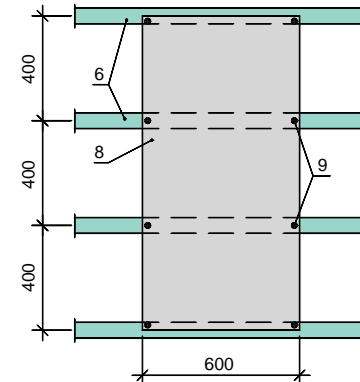
Befestigung von 600x1200 Platten mit 8 Schrauben
