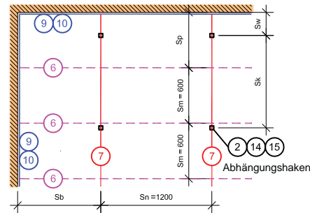
Profilanordnung für die Montage von 595x1195 mm Platten d) S_n=1200 mm
