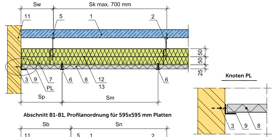
Abschnitt A1-A1, Profilanordnung für 595x595 mm Platten
