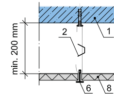
Montagehöhe - Schnellabhängung
